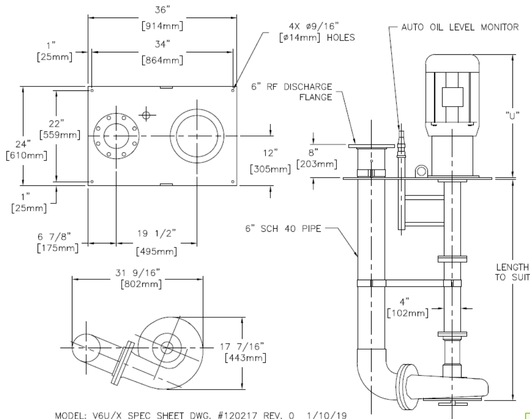
MODEL: V6U/X SPEC SHEET DWG. #120217 REV. 0 1/10/19
